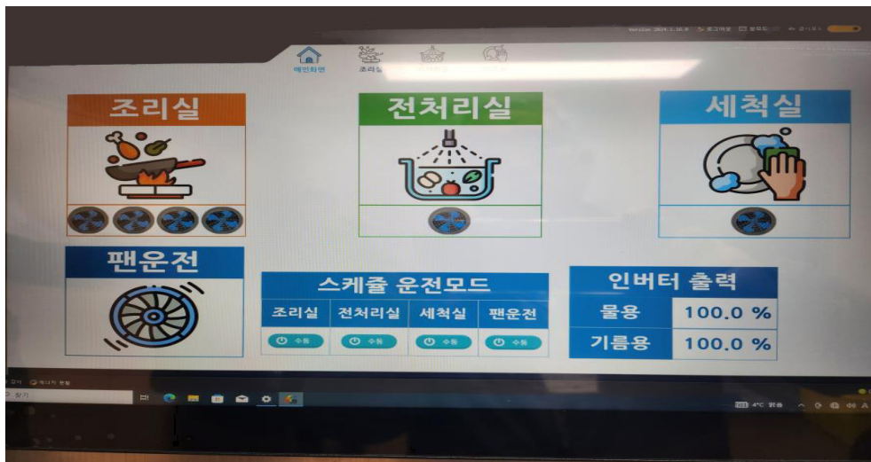
〈멤퍼조작화면-초기화면〉
