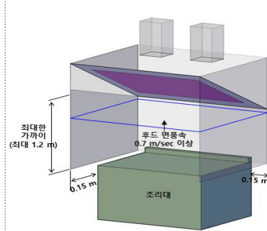
<사이드패널 설치>
