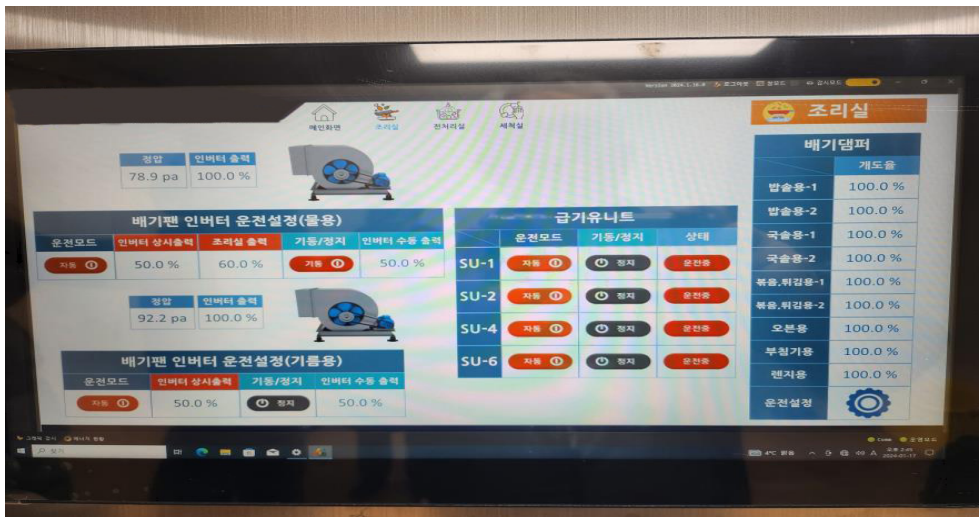
〈멤퍼조작화면-조리실〉
